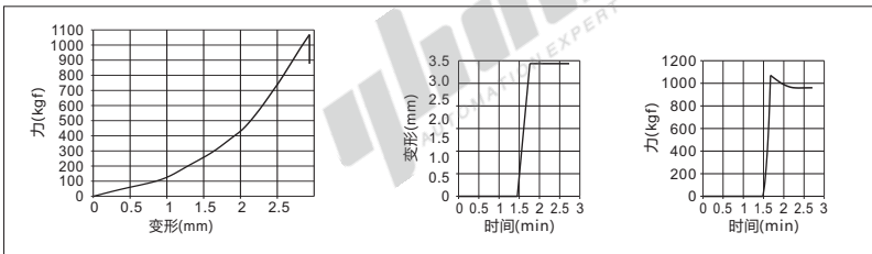
● 承载力试验 (测验型号: WAL01-D120-M24-L125)
