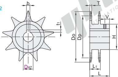
链轮 VLW02
